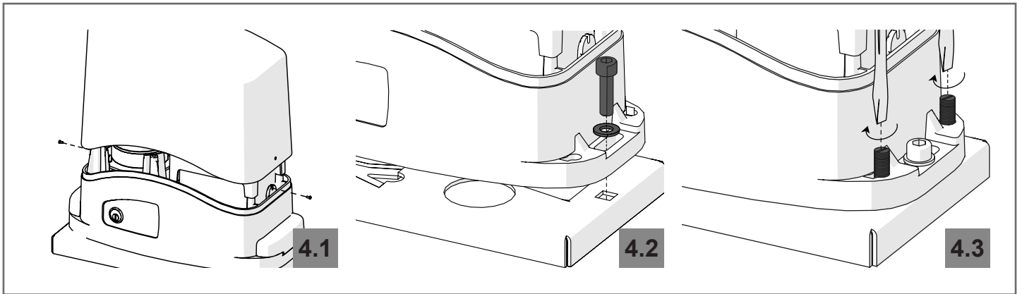
Fig. 5 EN - Rack assembling
