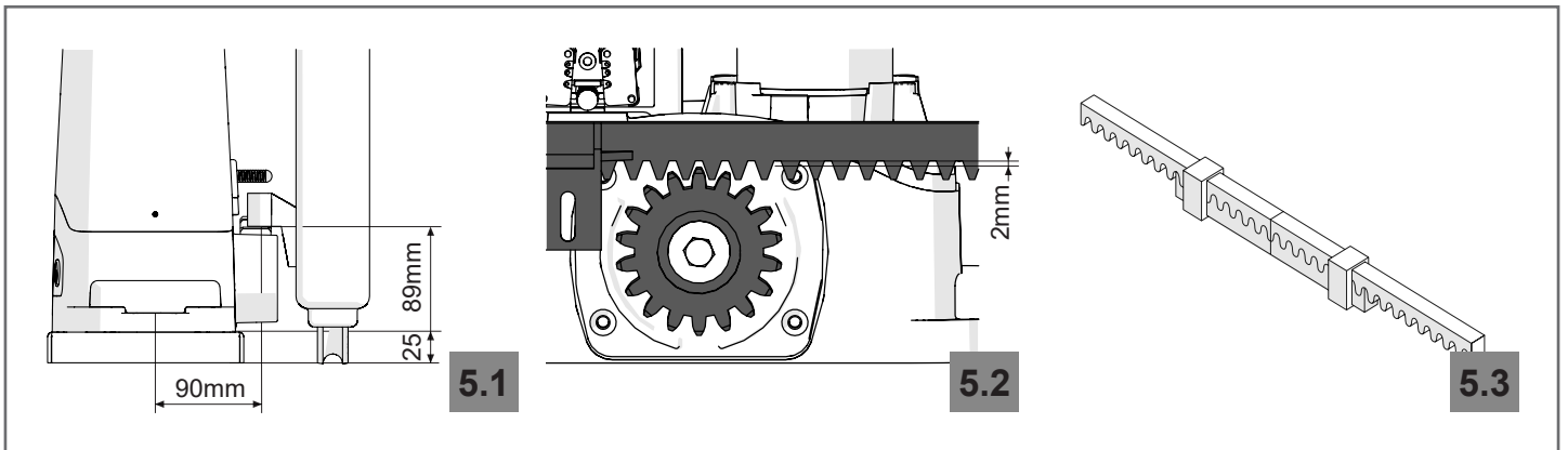
Fig. 6 EN - Limit switch fixing
